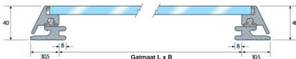
Profiel Standaard luik zonder flens
