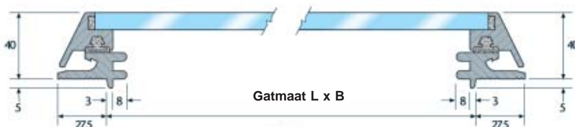
Profiel Standaard luik met flens
